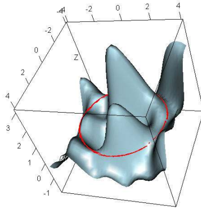
Figure 1: Réalisation d’un processus centré de covariance K nul sur le cercle
