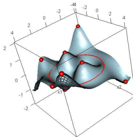
Figure 2: Meilleur prédicteur d’un krigeage avec condition sur le cercle
