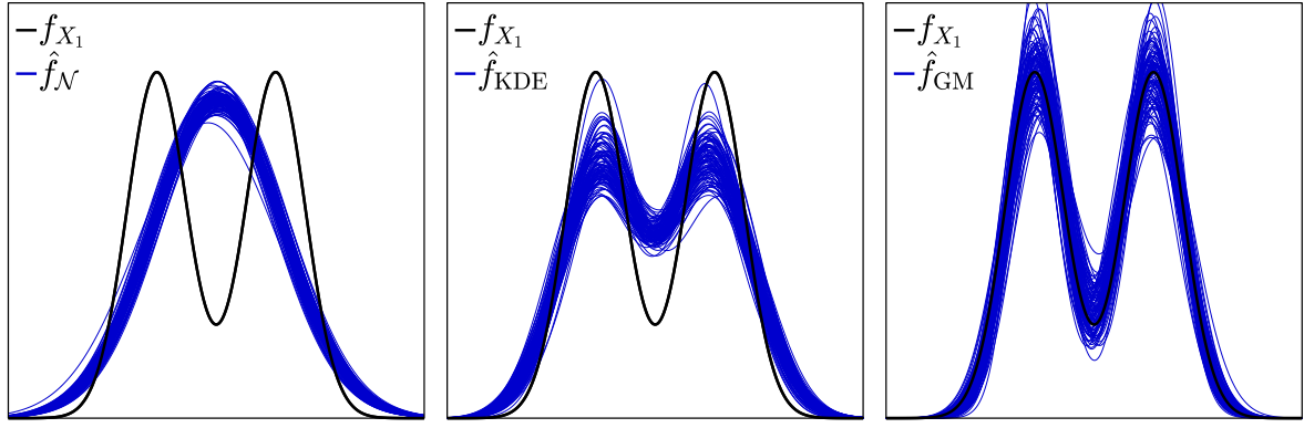
(a) Calibration MV d'une loi unimodale. (b) Approche non-paramétrique. (c) Calibration EM d'une loi bimodale.
